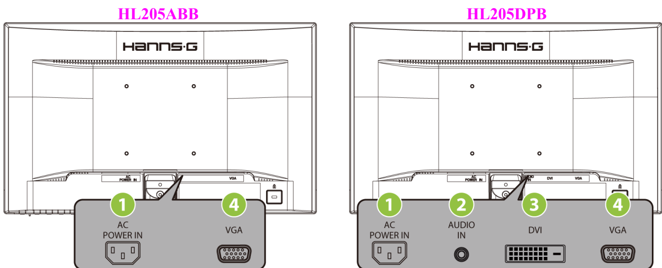
Εικόνα 2 Σύνδεση καλωδίων
