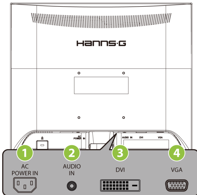
Obrázek 2. Propojovací kabely
