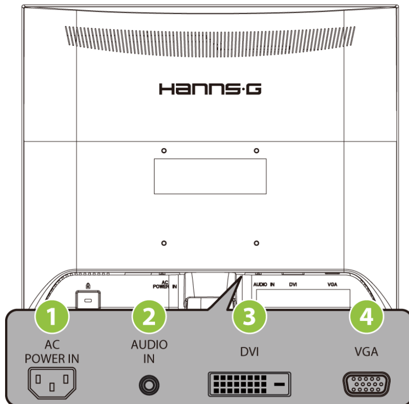
ABBILDUNG 2. ANSCHLISSEN AN EINEN PC
