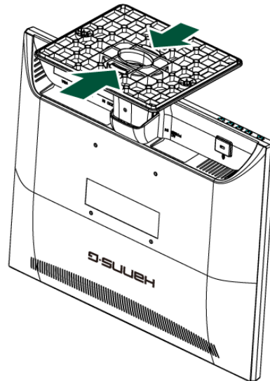
Εικόνα 1 Εγκατάσταση και απομάκρυνση της βάσης
