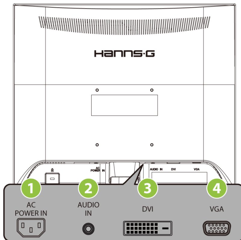
Afbeelding 2. AANSLUITEN OP EEN PC
