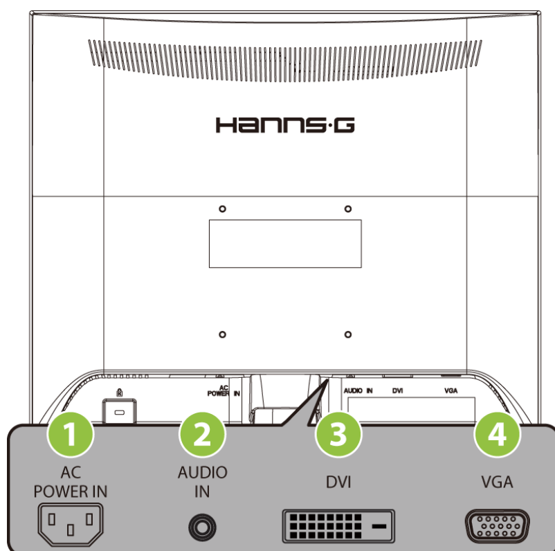
Ilustracja 2 Podłączenia kabli
