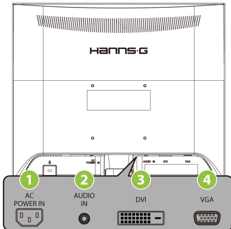
Bild 2. Koppla kablarna
