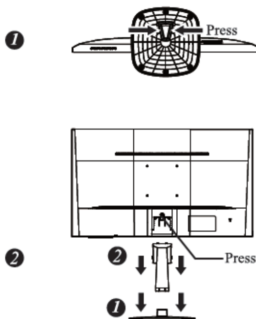
ABBILDUNG 1. INSTALLIEREN UND ENTFERNEN DES STÄNDERS
