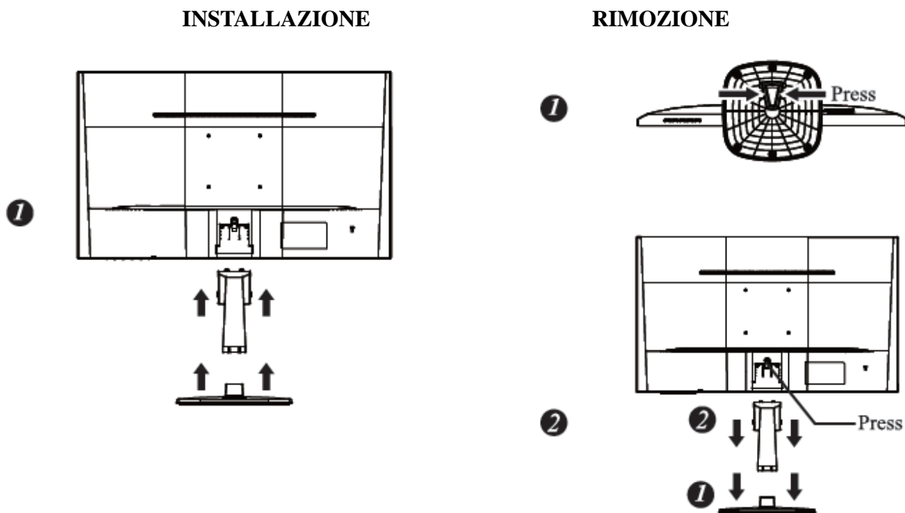
Figura.1. Installazione e Rimozione della Base
