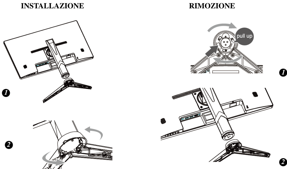
Figura.1. Installazione e Rimozione della Base
